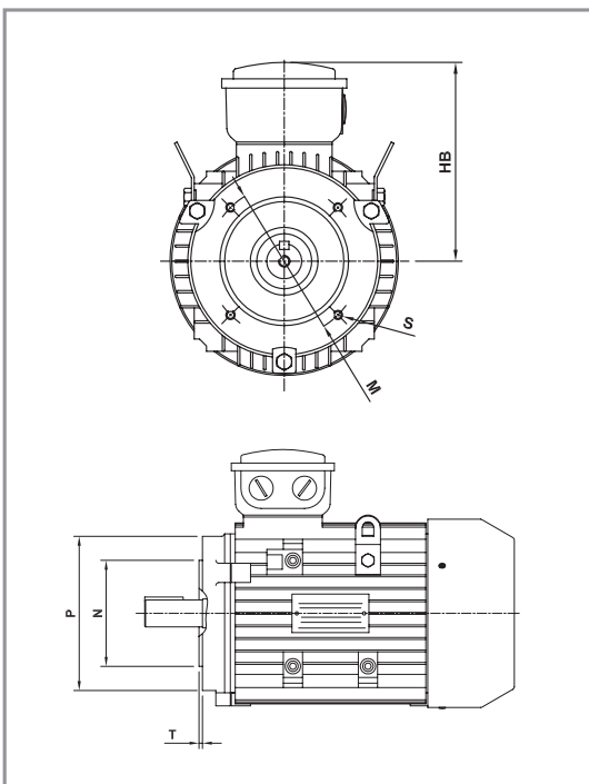
FACE MOUNT B14A (IM3601)
