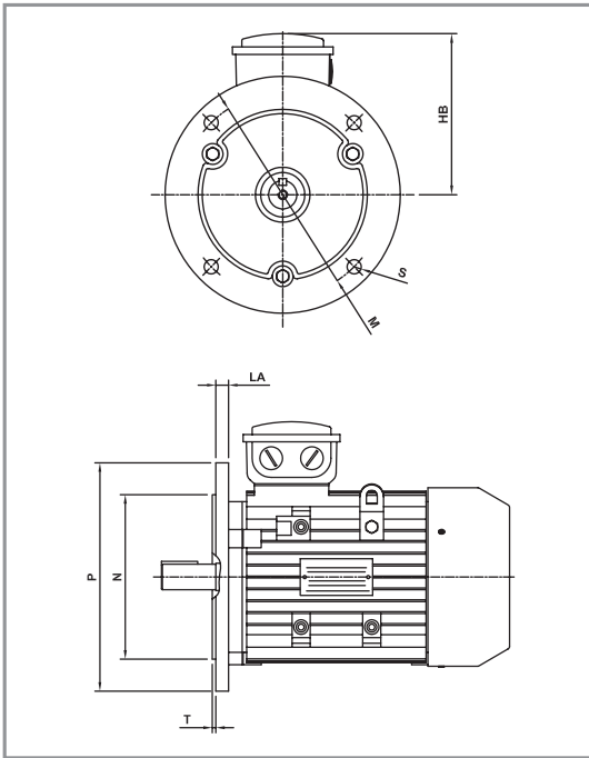
FLANGE MOUNT B5 (IM3001)
